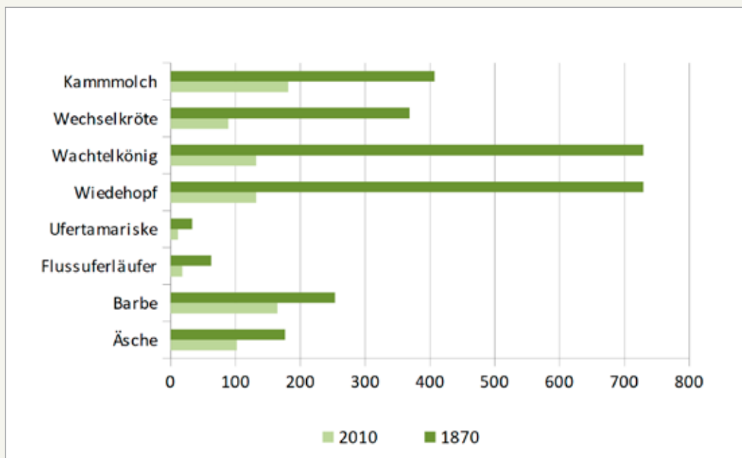
Abb. 2: Rückgang geeigneter Lebensräume für ausgewählte gefährdete Arten an großen Flüssen von 1870 bis 2010. Daten: Revital. Grafik: WWF. Angaben in km².
