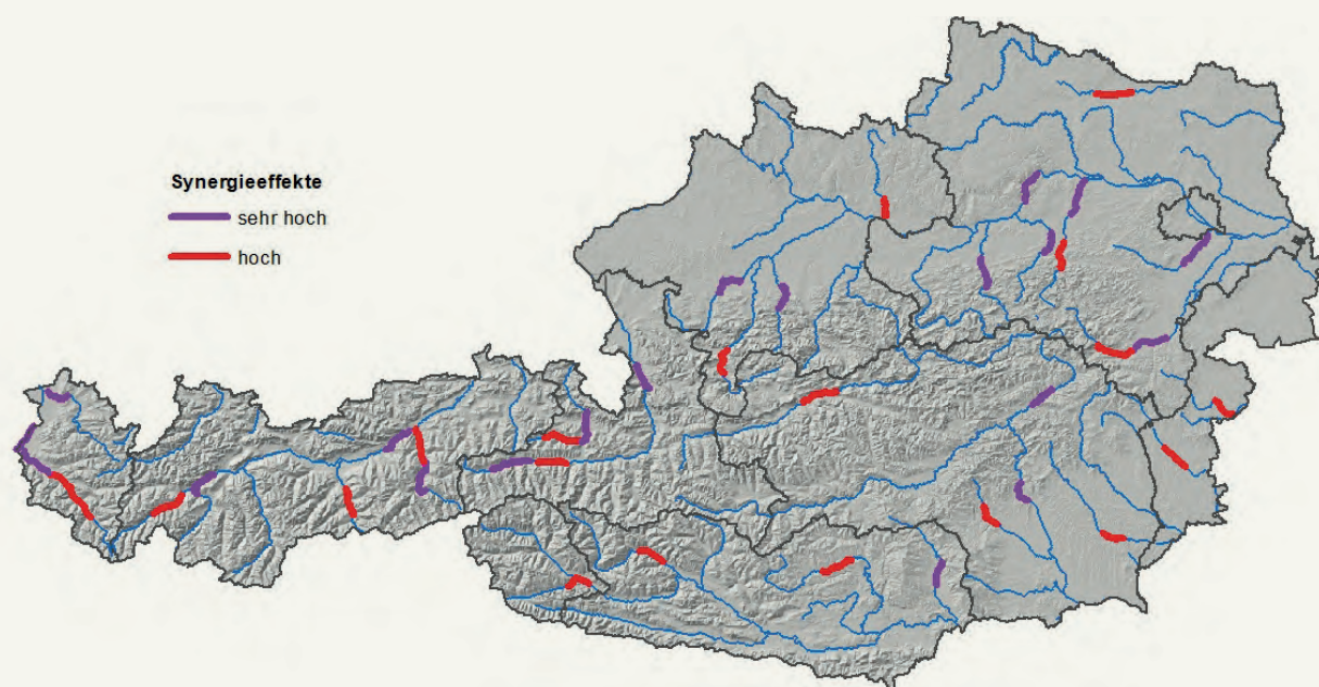
Abb.8: Übersicht Flussstrecken mit Synergieeffekten aus Ökologie und Hochwasserschutz
